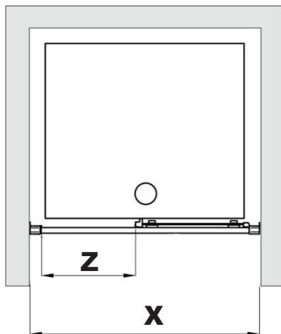
,Tabela 1. Dimenzije ulaznog otvora kabine
