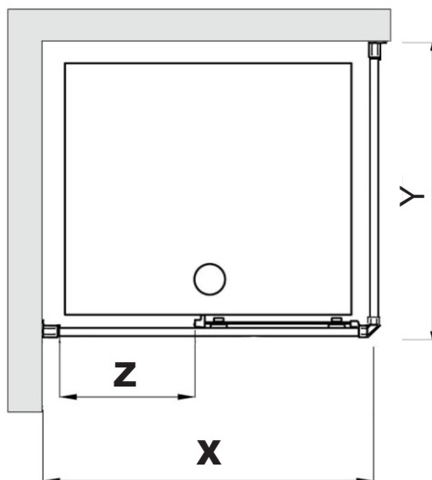
,Tabela 1. Dimenzije ulaznog otvora kabine
